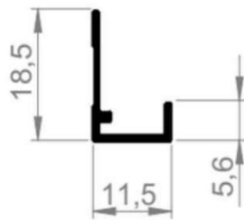
TP-001 TRILHO J RETO REBAIXADO EMBALAGEM 10 BRS
