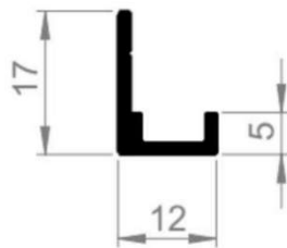
TP-003 TRILHO J RETO COM ABA EMBALAGEM 10 BRS
