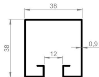
TP-381 TRILHO PANTOGRAFICO 38 X 38 COMERCIAL EMBALAGEM 10 BRS
