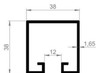
TP-383 TRILHO PANTOGRAFICO 38 X 38 EXTRA EMBALAGEM 10 BRS
