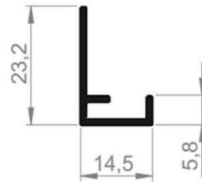
TP-002 TRILHO J RETO EMBALAGEM 10 BRS
