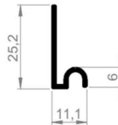
TP-004 TRILHO H ABALADO EMBALAGEM 10 BRS
