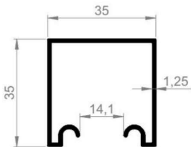
TP-353 TRILHO PANTOGRAFICO 35 X 35 EXTRA EMBALAGEM 10 BRS
