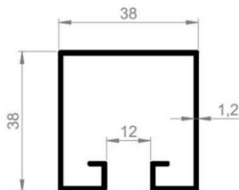
TP-382 TRILHO PANTOGRAFICO 38 X 38 REFORÇADO EMBALAGEM 10 BRS
