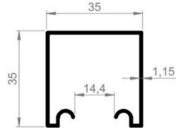
TP-352 TRILHO PANTOGRAFICO 35 X 35 REFORÇADO EMBALAGEM 10 BRS
